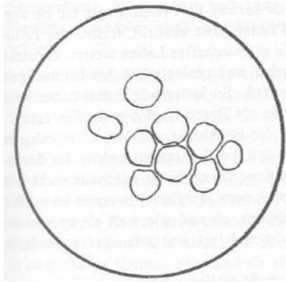
Illustration 31 Levure rachitique qui s'est formée dans la sphère du vide (sous l'éviction du rayonnement structural)
