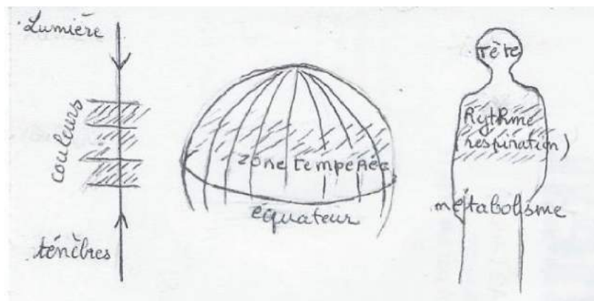
Illustration 13. Lumière - Couleur - Ténèbres - Pôle - zone tempérée ( saisons ) équateur - tête - rythme respiratoire - métabolisme : comme résultat de l'action entre deux polarités.
