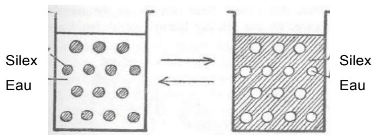
Illustration 41. Passage de l'état hydrosol à l'état hydrogel (gélatine)
