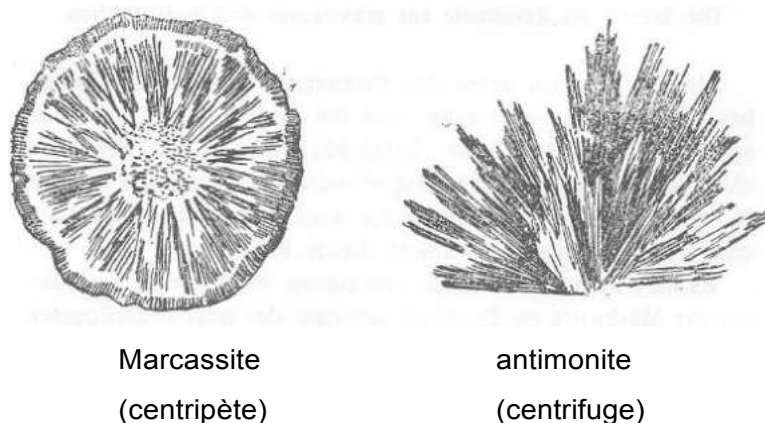
Illustration 59: Forces formatrices rayonnant vers l'intérieur et vers l'extérieur.
