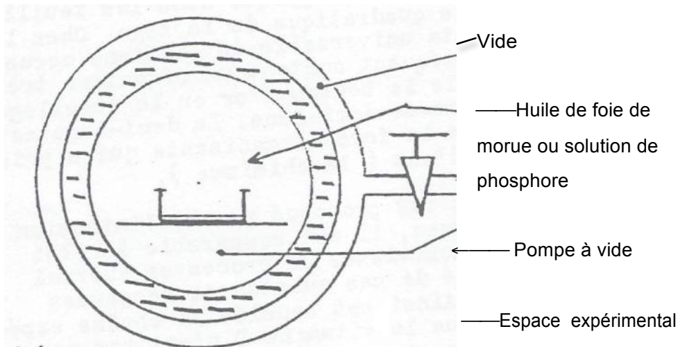
Illustration 25 : Représentation illustrée du montage expérimental destiné à supprimer l'action du vide (le rachitisme.) grâce à l'action rayonnante d'une sphère de foie de morue ou d'une sphère de phosphore.
