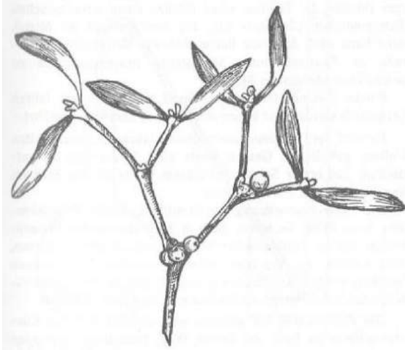
Illustration 34 : La structure dichotomique du gui (rythme à 2 temps)
