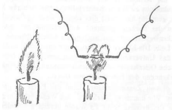
Illustration 11. Flamme d'une bougie. Rétroversion de la flamme par l'étincelle d'induction; formation d'un squelette de charbon entre les deux pôles.
