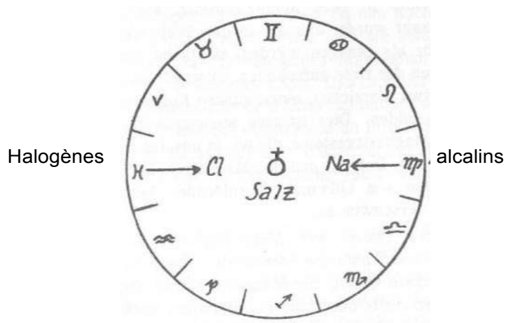
Illustration 50 - Alcalins et halogènes en tant que précipités des forces venant de la Vierge et des Poissons. Lire au milieu : sel.
