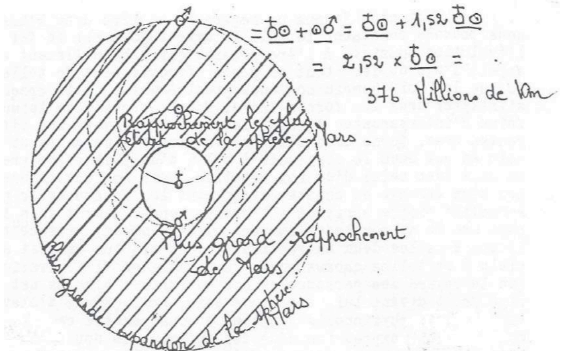
Illustration 60. Inspiration et expiration (Respiration) de la sphère Mars.
