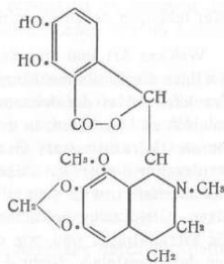
nornacotine méthylique
