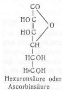
Acide hexuron ou acide ascorbique
