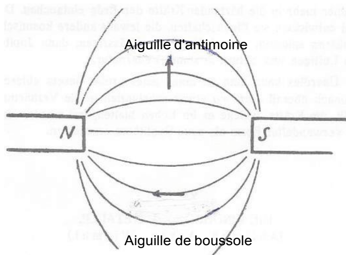
Illustration 66. Le magnétisme du fer et le diamagnétisme (anti magnétisme) de l'antimoine.
