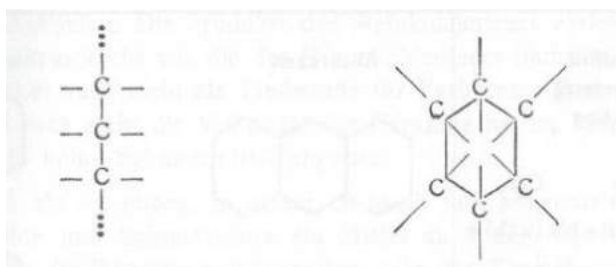
Chaîne ouverte de la paraffine
