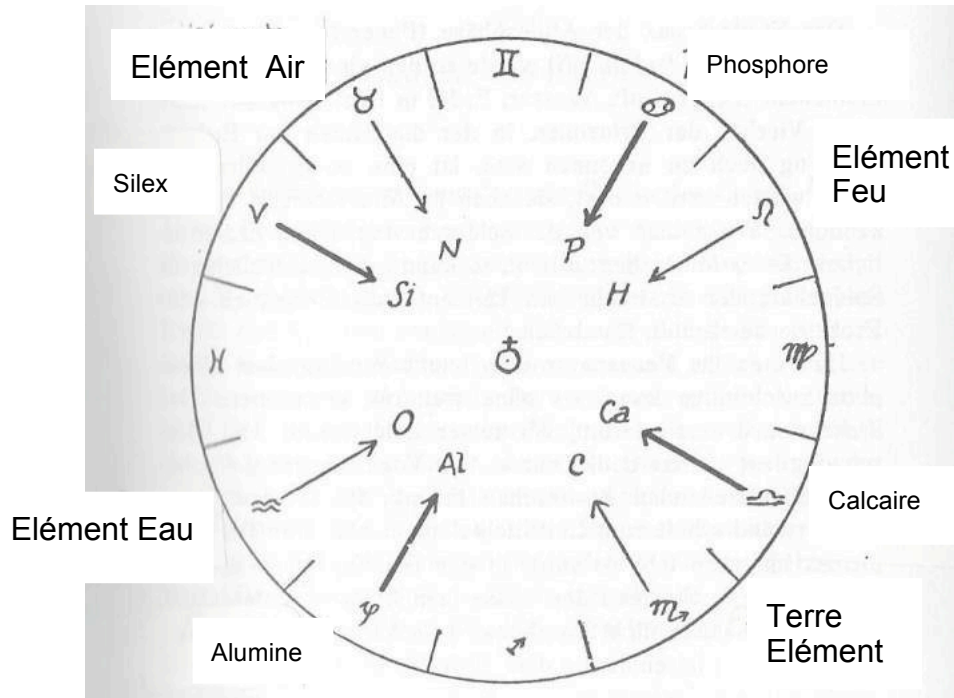
Illustration 49 La croix minéralogique à côté de la croix atmosphérique.
