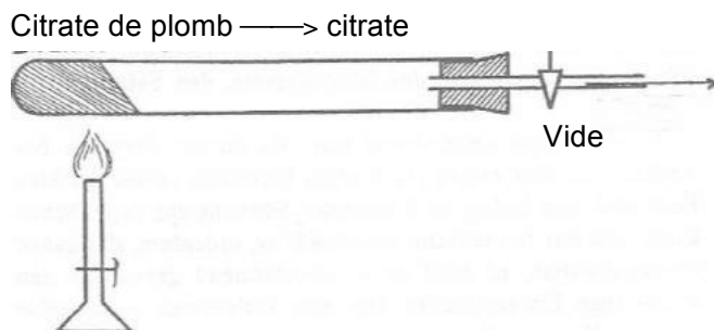
Illustration 56. Montage expérimental pour la fabrication du plomb pyrophorique.
