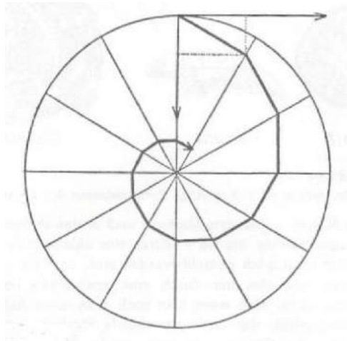
Illustration 57 : La spirale comme résultante des forces sphériques et radiales
