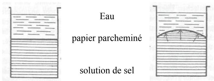
Illustration 33. La pression osmotique exercée par une substance diluée sur les parois du vase.
