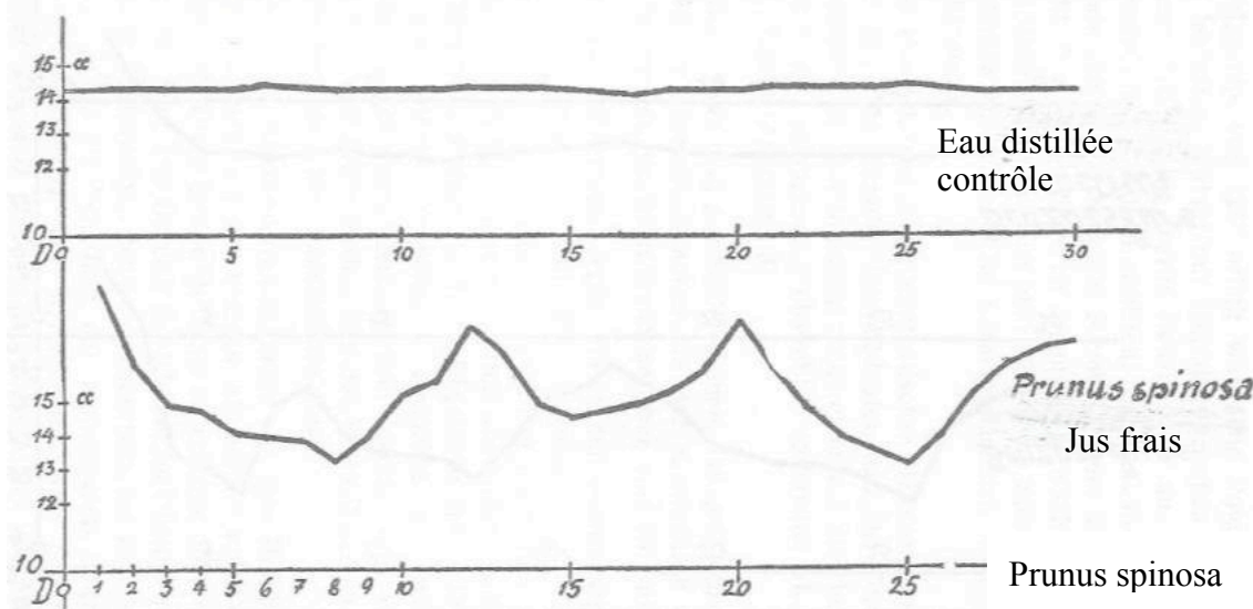
Illustration 36. Courbe de potentialité du prunus Spinoza (prunelier à épines noires)
