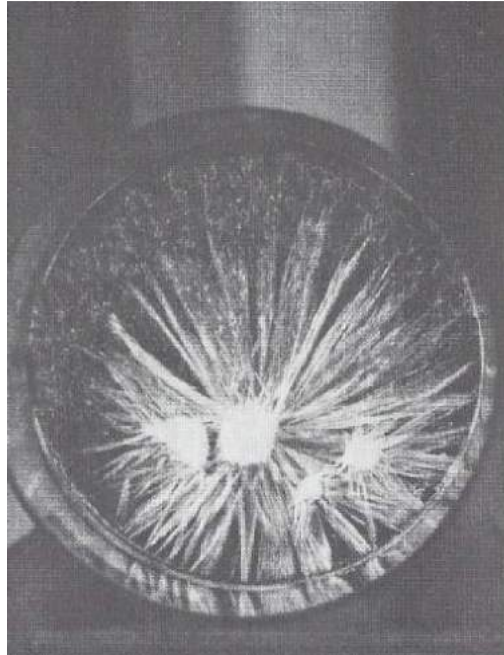
Illustration 22 : Cristallisation dans la sphère vide. Quartier de lune et demi-lune comme "formation rachitique" ; l'auréole cristallise d'abord au moment de l'élimination du vide.
