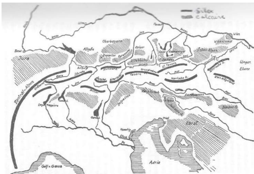
Illustration 40. Silice et calcaire comme substances de construction des Alpes (Alpes centrales, Alpes calcaires du Sud et du Nord)
