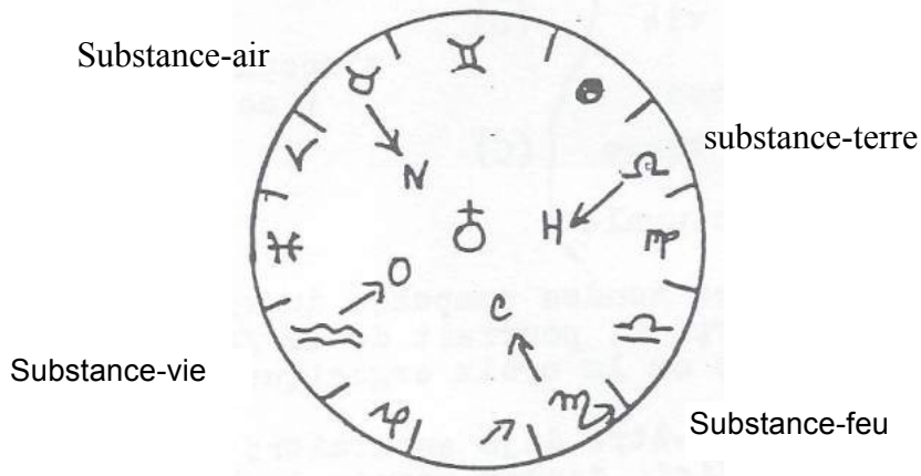
Illustration 14 : La croix des atmosphères
