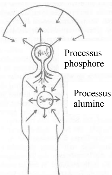
Illustration 47. Nerfs et sang comme manifestation du processus alumine-phosphore
