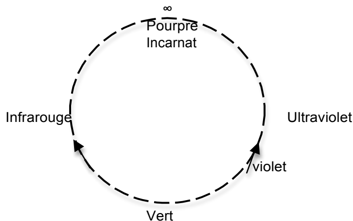
Illustration 20. Le cercle des couleurs de l'Univers.
