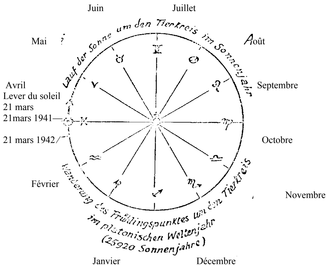
Illustration 9. Représentation schématique des mouvements du Soleil : année solaire et année des mondes dite platonicienne.
