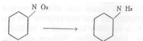
Nitrobenzène
